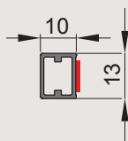
DIV-204 Cross profile Querprofil Travesaño Traverse
