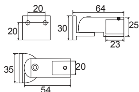
B-164 • Jungtis 135° Ø19 mm vamzdžiui. • 135° connector for 19 mm tube Forged brass.
