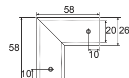
B-173 • Reguliuojama jungtis Ø 19 mm vamzdžiui. • Adjustable connector for Ø 19 mm tube.
