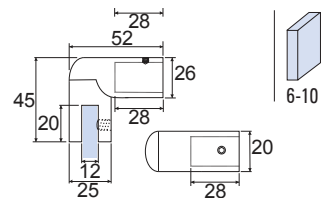
B-165 • Jungtis 90° Ø19 mm vamzdžiui. • 90° connector for 19 mm tube.
