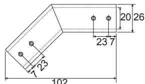
B-184 • Sieninis galas 45° Ø 19 mm stiklo laikymo strypams. • Wall fixing bar 45° end for Ø 19 mm tube.
