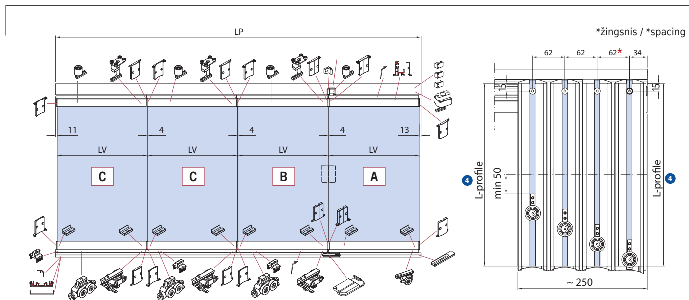
Stiklo prispaudimo profilis Glass profile
