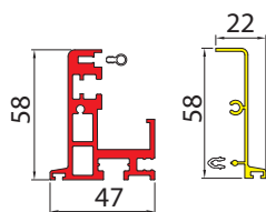
Stiklo prispaudimo profilis Glass profile
