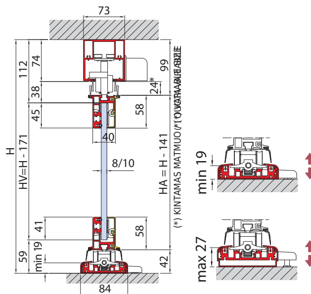
REGULIUOJAMAS APATINIS KREIPIKLIS Adjustable floor channel
