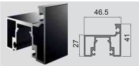
TP-150 Durų stakta / Door jamb
