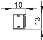
DIV-204 PASIRINKTINAI DIV-204 OPTIONAL CROSS PROFILE SKERSINIS
