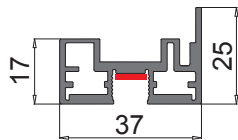
④ DIV-104 VERTIKALUS PROFILIS (dvivėrės varstomos durys, priešplokštės pusė) VERTICAL PROFILE (double hinged door, strike plate side) VERTIKALUS PROFILIS (dvivėrės durys, priešplokštės pusė) VERTICAL PROFILE (double door - strike side)
