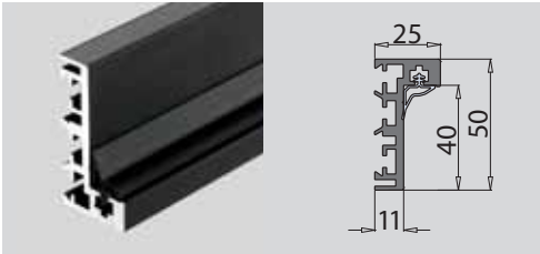
P-030/P-031 Durų stakta / Door jamb
