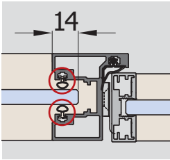
B-146 Glass gaskets mm 8/10 mm Stiklo tarpinės mm 8/10 mm
