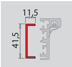
Optional wall profile for adjustment P-033 Pasirinktinai: sieninis reguliavimo profilis P-033
