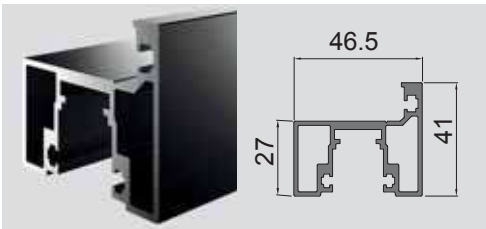
TP-150 Durų stakta / Door jamb
