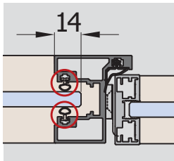
B-146 Glass gaskets mm 8/10 mm Stiklo tarpinės mm 8/10 mm
