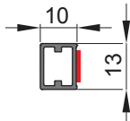
DIV-204 OPTIONAL / DIV-204 PASIRINKTINAI CROSS PROFILE SKERSINIS
