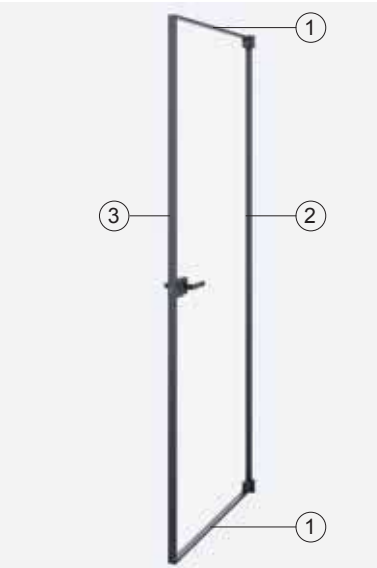
① DIV-103 HORIZONTAL TOP AND BOTTOM PROFILE HORIZONTALUS VIRŠUTINIS IR APATINIS PROFILIS
