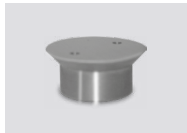
TA-011/10MA TA-011/12MA • Nerūdijančio plieno taškinis laikiklis su juoda nailono tarpine, Ø 40 mm x H 16,4 mm, vidinis sriegis M10 arba M12, skylė stiklė 31 - 31,5 mm su nuožula 5x45°. • Point holder in stainless steel with gasket, Ø 40 mm x H 16,4 mm, thread M10 or M12, glass hole 31 - 31,5 mm with countersunk 5x45°.
