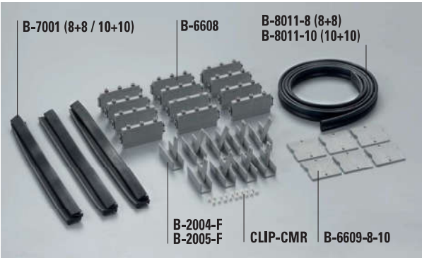
B-SET-7020-8 / B-SET-7020-10 • Laikiklių ir tarpinių komplektas, dvigubas reguliavimas • Set clamps and gaskets, double regulation
